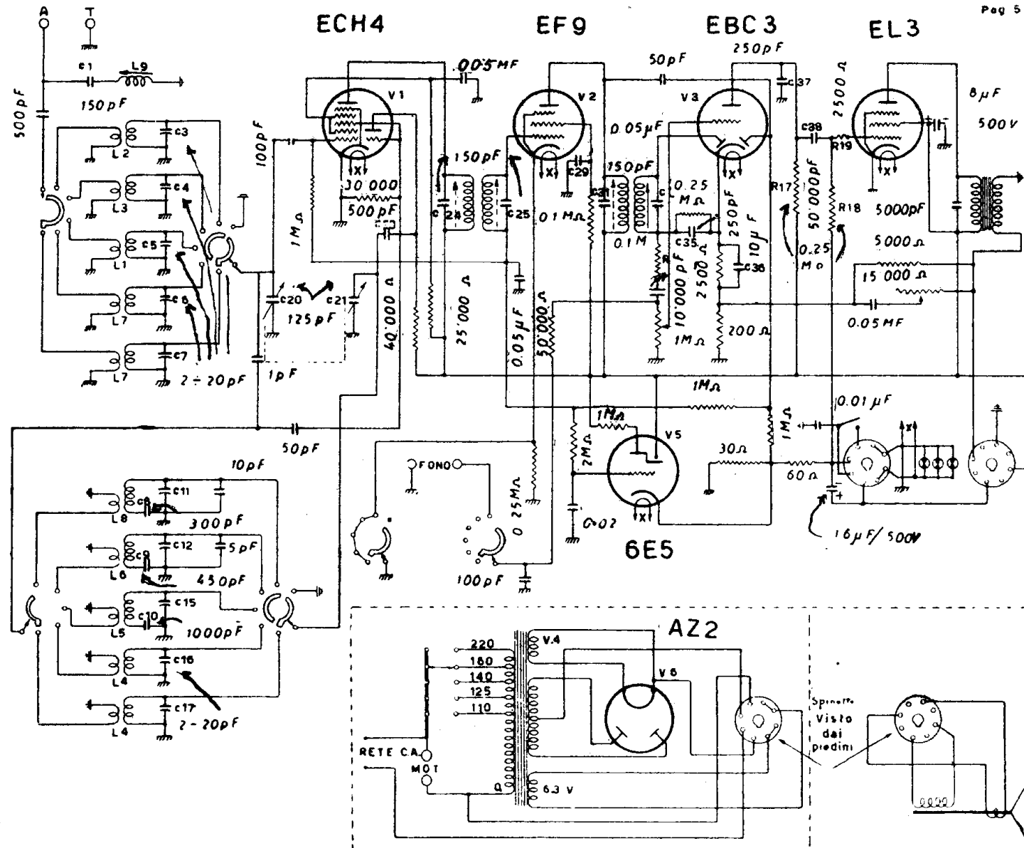
ALLOCCIO BACCHINI - Modd. 619 e 629 - Medie divise e tre corte. Media frequenza 465 kc. Finale: placca 240 V, schermo 250 V, catodo 6 V. Altre placche 250 V. Corrente totale 55 mA.
